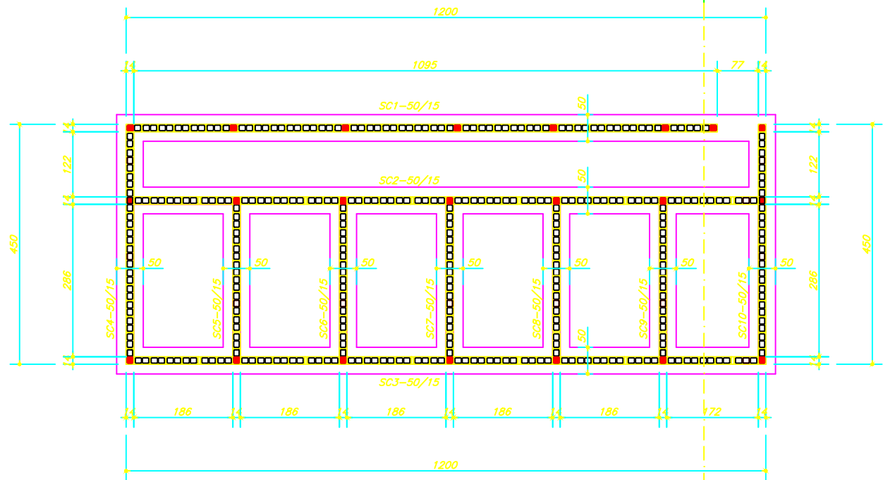
ARQUIBANCADA - FUNDAÇÃO
