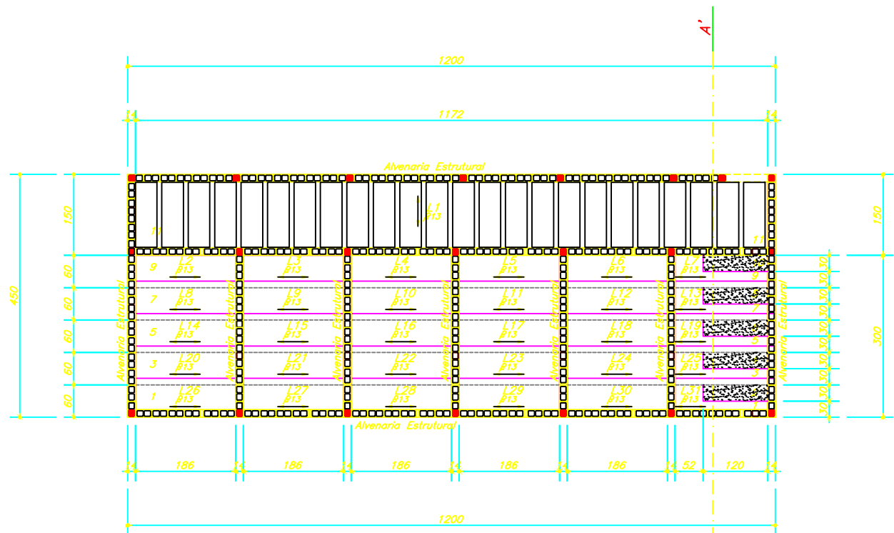
ARQUIBANCADA - LAJES
