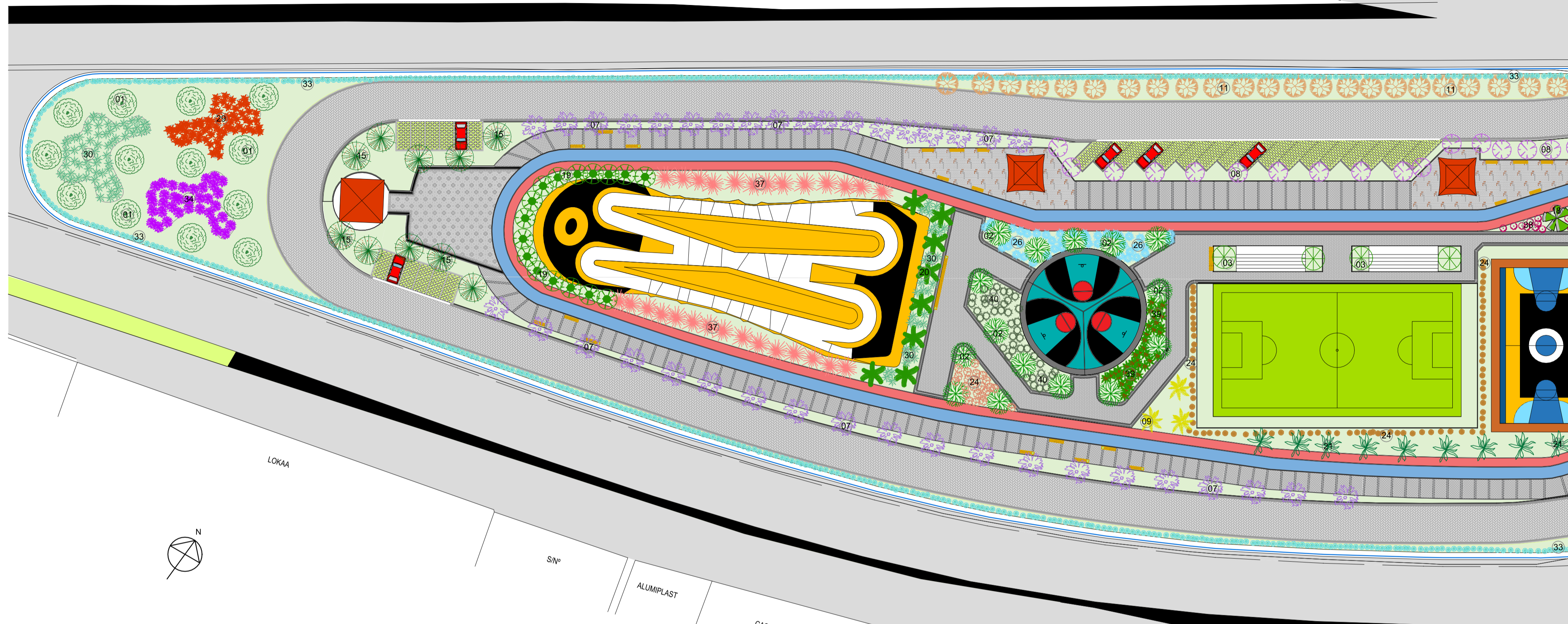
01 PLANTA BAIXA TRECHO 01 - PLANTIO ESC. 1/500
