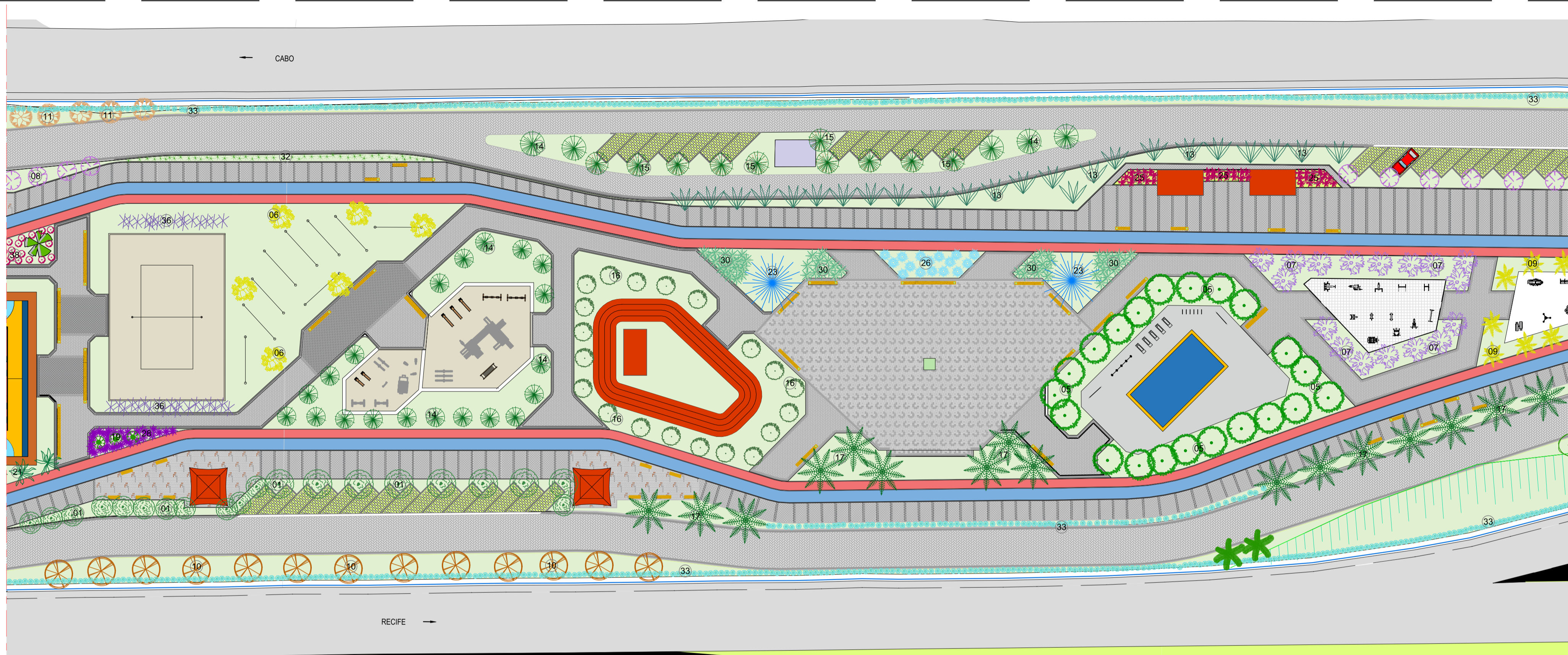
01 PLANTA BAIXA TRECHO 02 - PLANTIO ESC. 1/500
