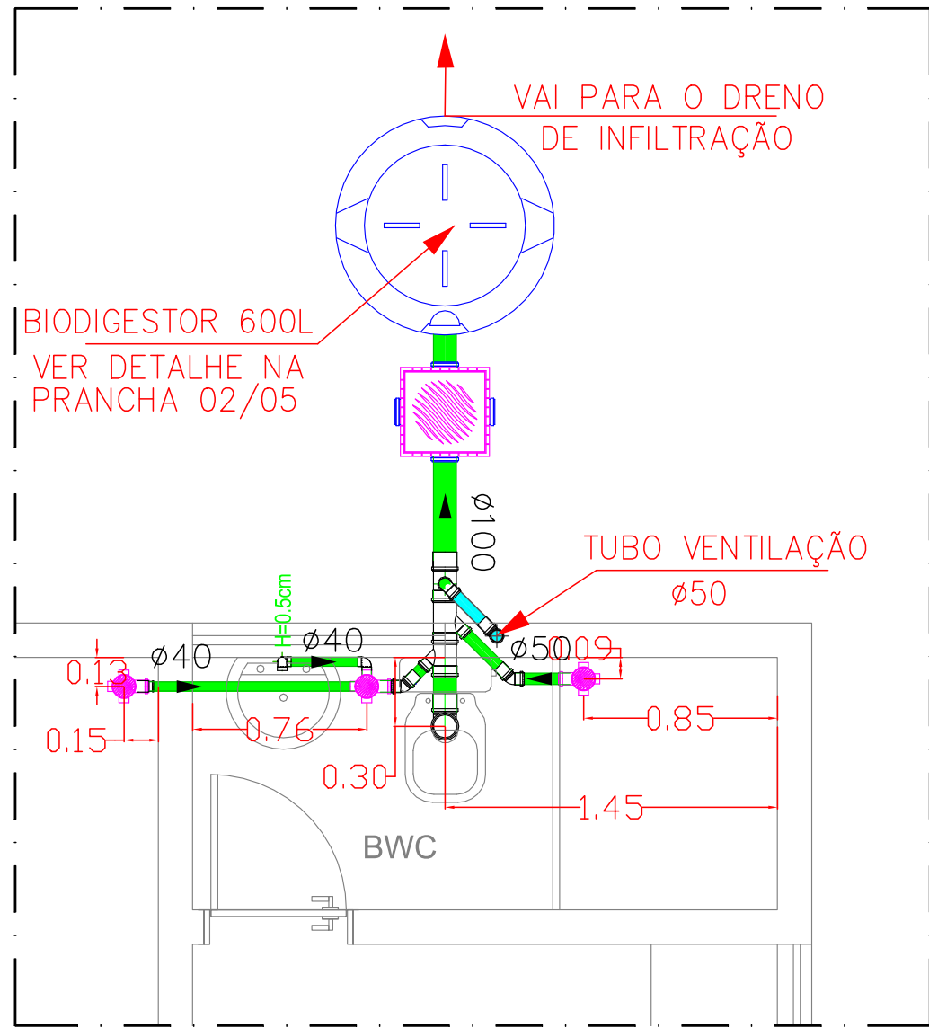
DETALHE - 06 POSTO MÉDICO / POLICIAL ESCALA: 1:20
