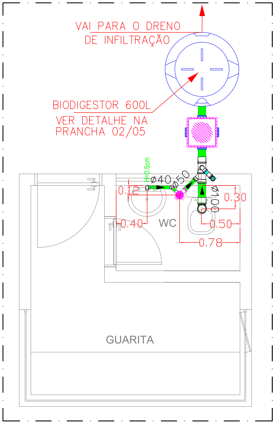
PLANTA BAIXA - ESGOTO GUARITA ESCALA: 1:20
