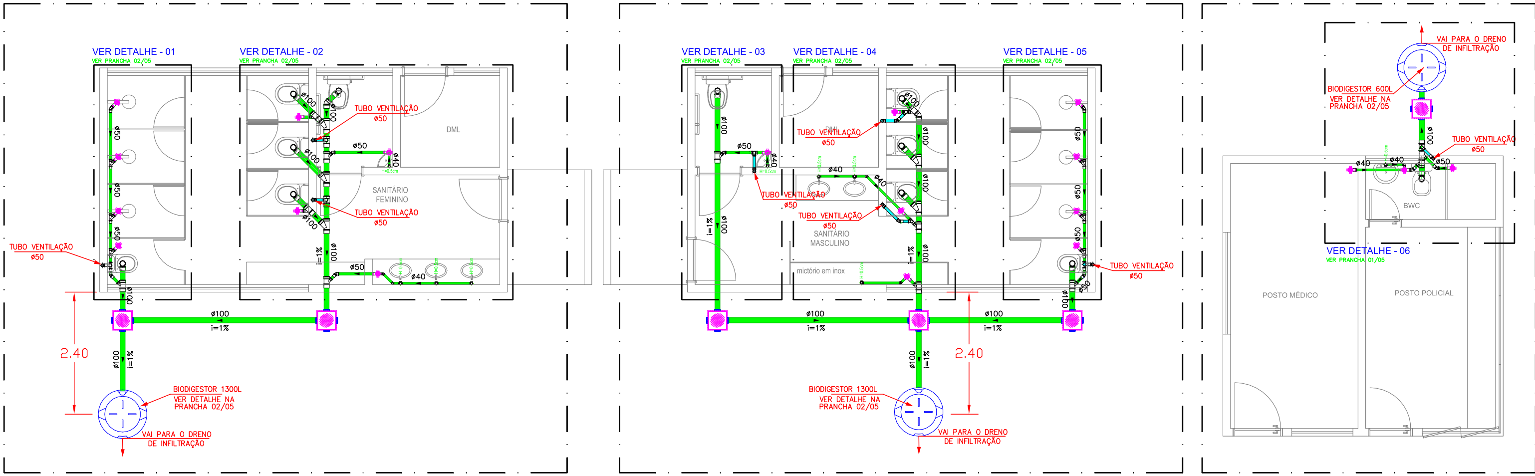
PLANTA BAIXA - ESGOTO SANITÁRIO FEMININO ESCALA: 1:50
