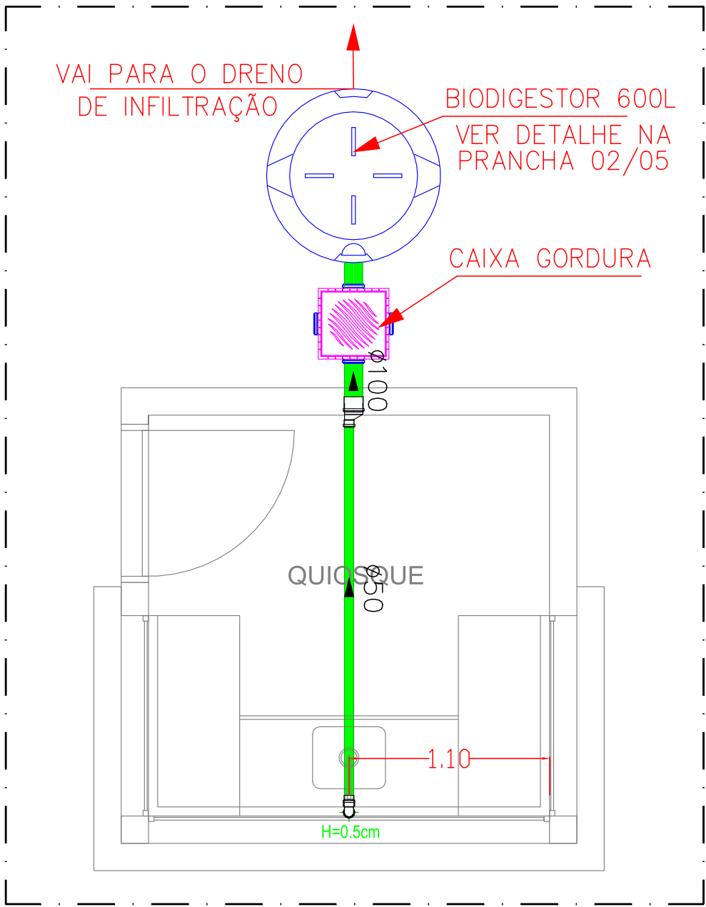
PLANTA BAIXA - ESGOTO QUIOSQUE ESCALA: 1:20
