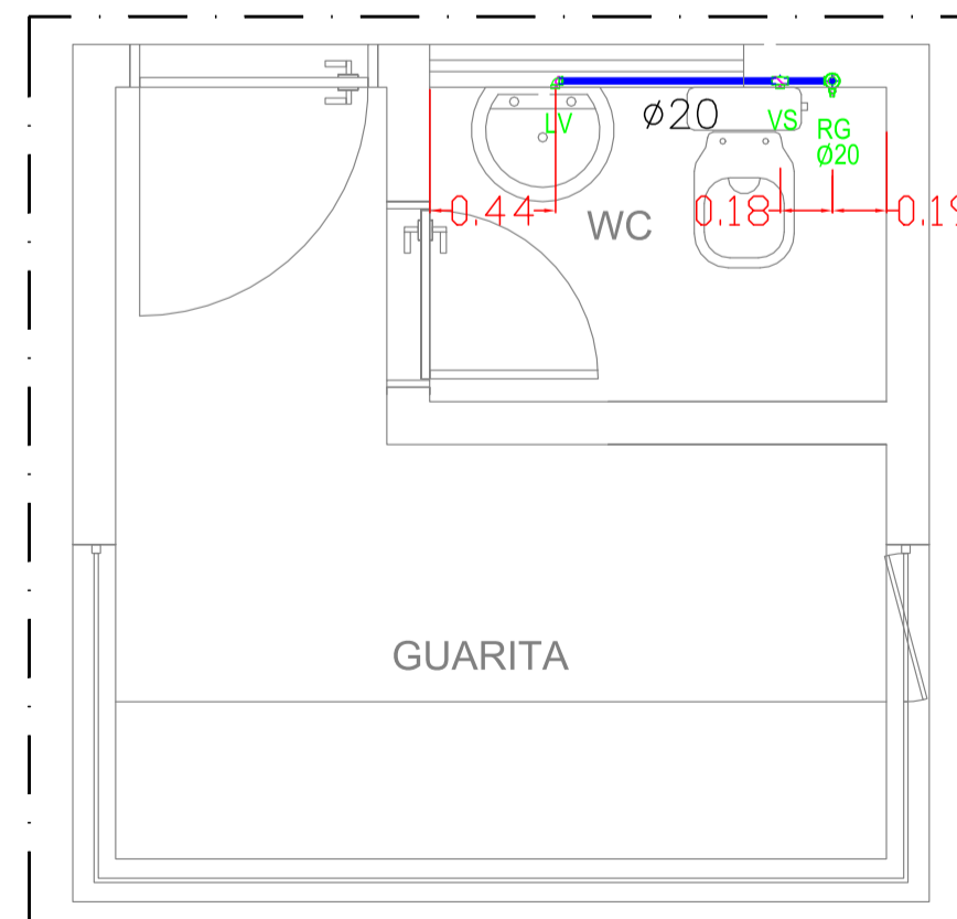
PLANTA BAIXA - ÁGUA FRIA GUARITA ESCALA: 1/20
