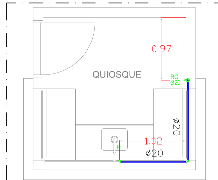
PLANTA BAIXA - ÁGUA FRIA QUIOSQUE ESCALA: 1/20
