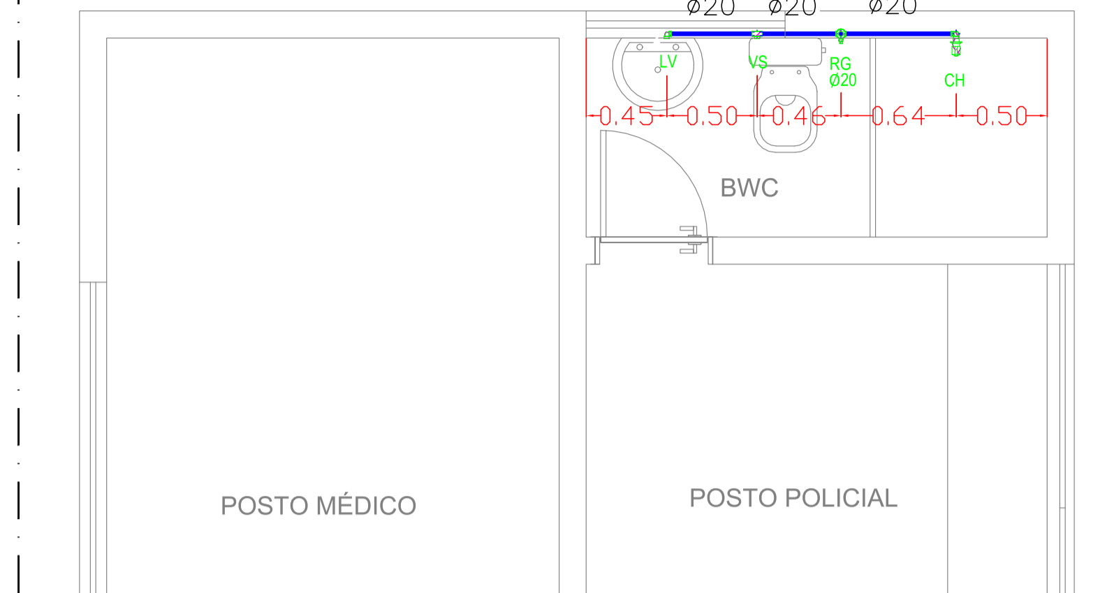
PLANTA BAIXA - ÁGUA FRIA POSTO MÉDICO / POLICIAL ESCALA: 1/20
