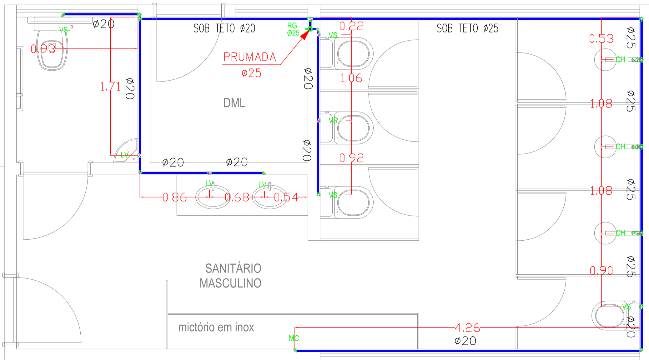
PLANTA BAIXA - ÁGUA FRIA SANITÁRIO MASCULINO ESCALA: 1/20
