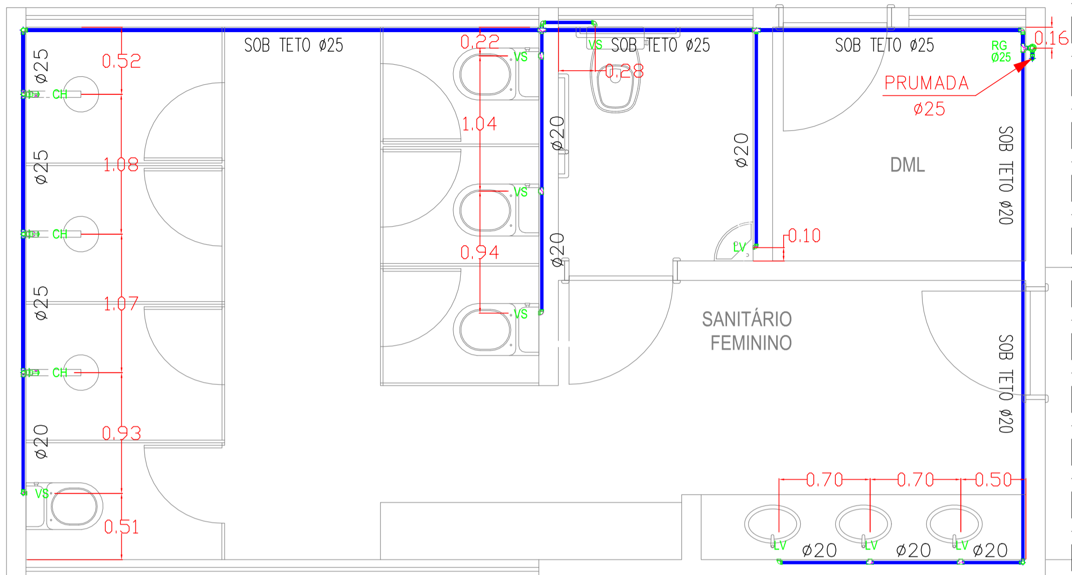
PLANTA BAIXA - ÁGUA FRIA SANITÁRIO FEMININO ESCALA: 1/20
