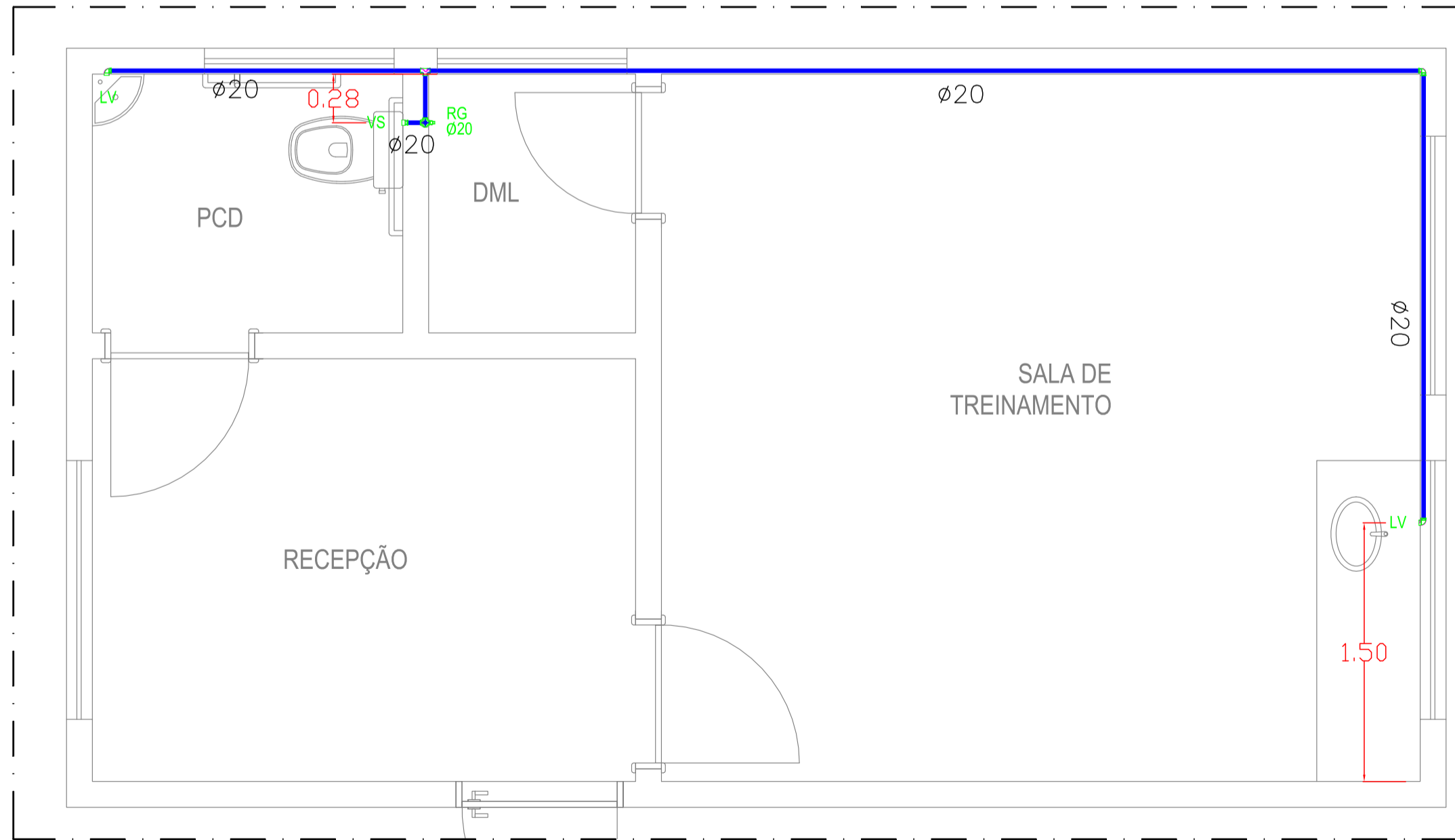
PLANTA BAIXA - ÁGUA FRIA CÃO TERAPIA ESCALA 1:20
