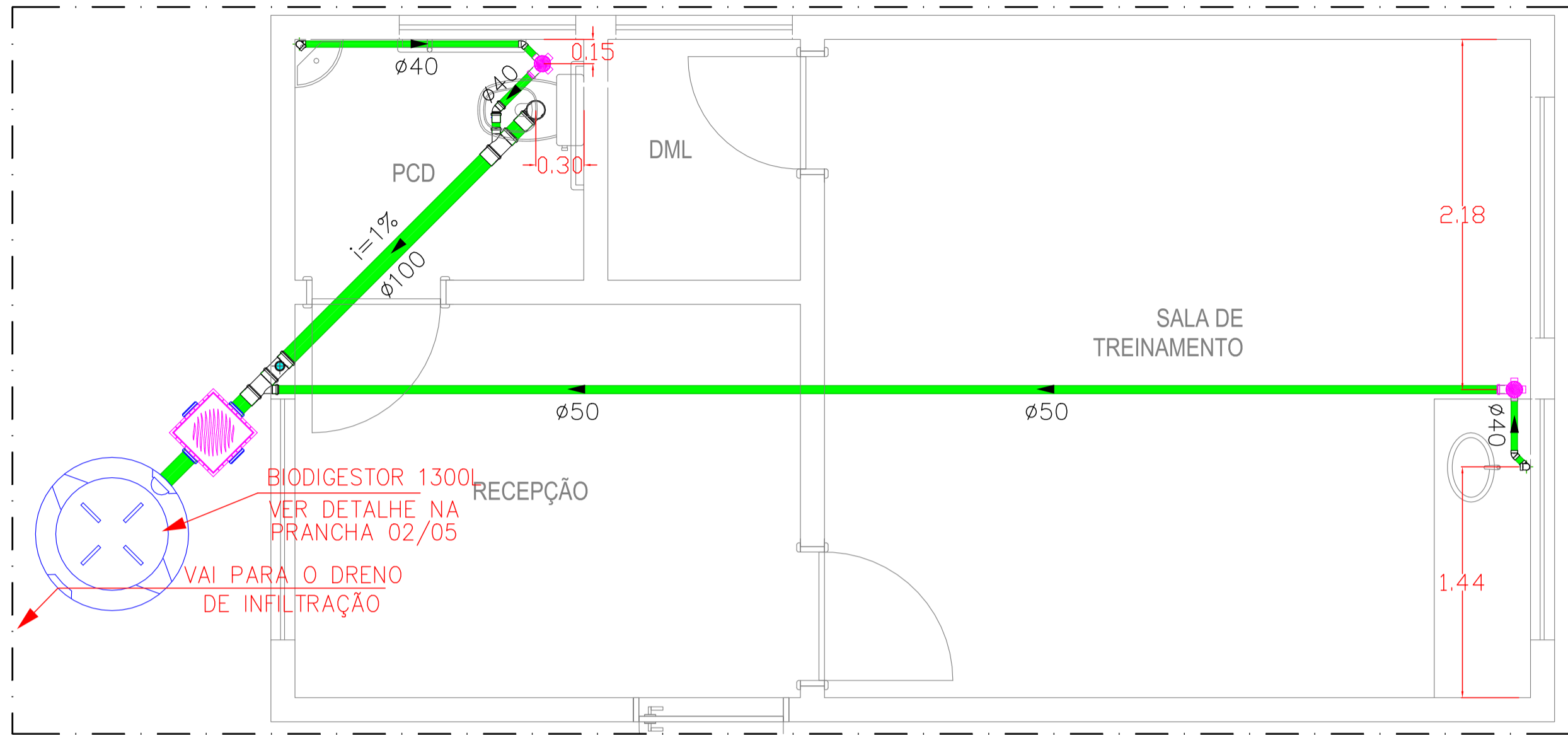
PLANTA BAIXA - ESGOTO CÃO TERAPIA ESCALA 1:20
